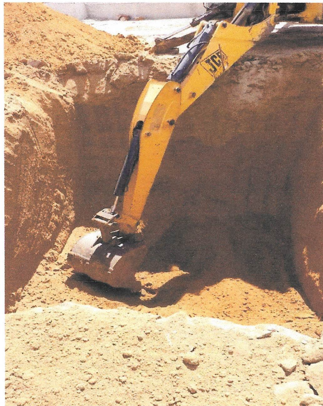
Foto 18 – ESCAVAÇÃO MECANIZADA PARA VIGA BALDRAME COM MINI- ESCAVADEIRA (INCLUINDO ESCAVAÇÃO PARA COLOCAÇÃO DE FÔRMAS). AF_06/2017
