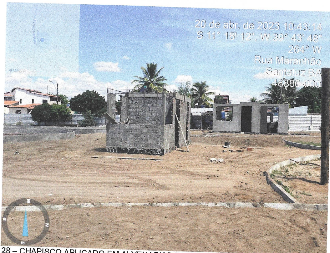
Foto 27 – EXECUÇÃO DE PASSEIO (CALÇADA) OU PISO DE CONCRETO COM CONCRETO MOLDADO IN LOCO, FEITO EM OBRA, ACABAMENTO CONVENCIONAL, ESPESSURA 6 CM, ARMADO. AF_07/2016
