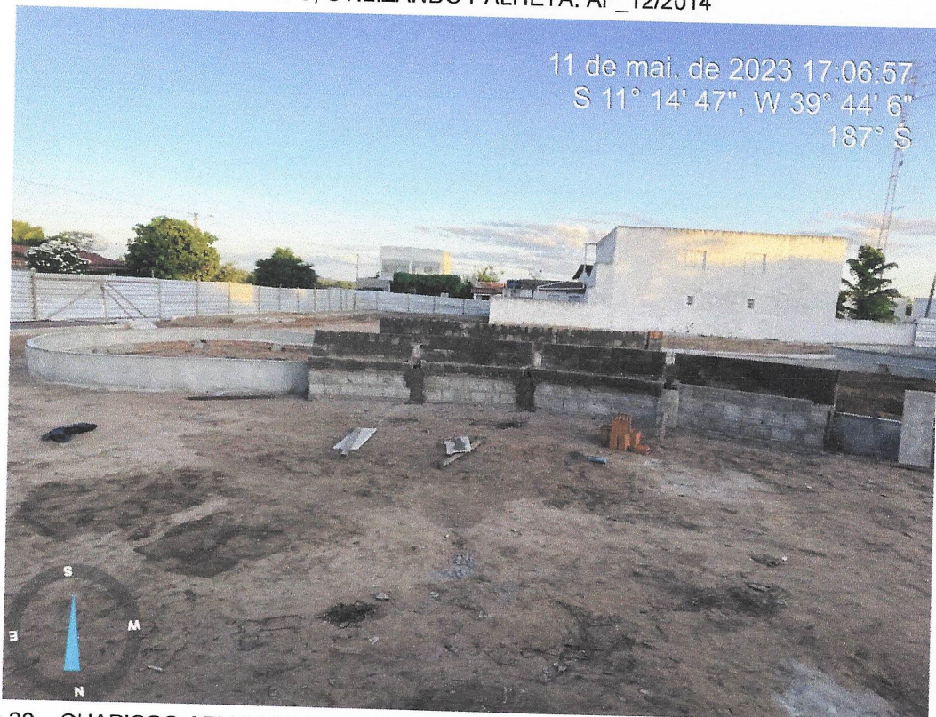
Foto 20 – CHAPISCO APLICADO EM ALVENARIA (COM PRESENÇA DE VÃOS) E ESTRUTURAS DE CONCRETO DE FACHADA, COM EQUIPAMENTO DE PROJEÇÃO. ARGAMASSA TRAÇO 1:3 COM PREPARO MANUAL.
