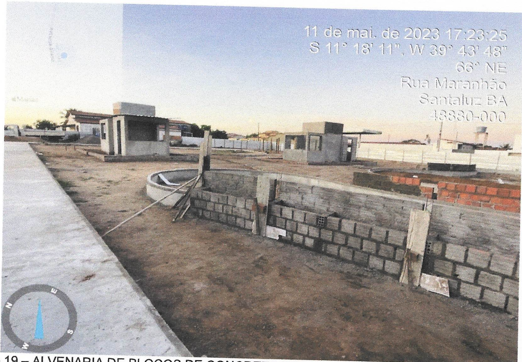
Foto 19 – ALVENARIA DE BLOCOS DE CONCRETO ESTRUTURAL 14X19X29 CM, (ESPESSURA 14 CM) FBK = 14,0 MPA, PARA PAREDES COM ÁREA LÍQUIDA MAIOR OU IGUAL A 6M 2 , SEM VÃOS, UTILIZANDO PALHETA. AF_12/2014
